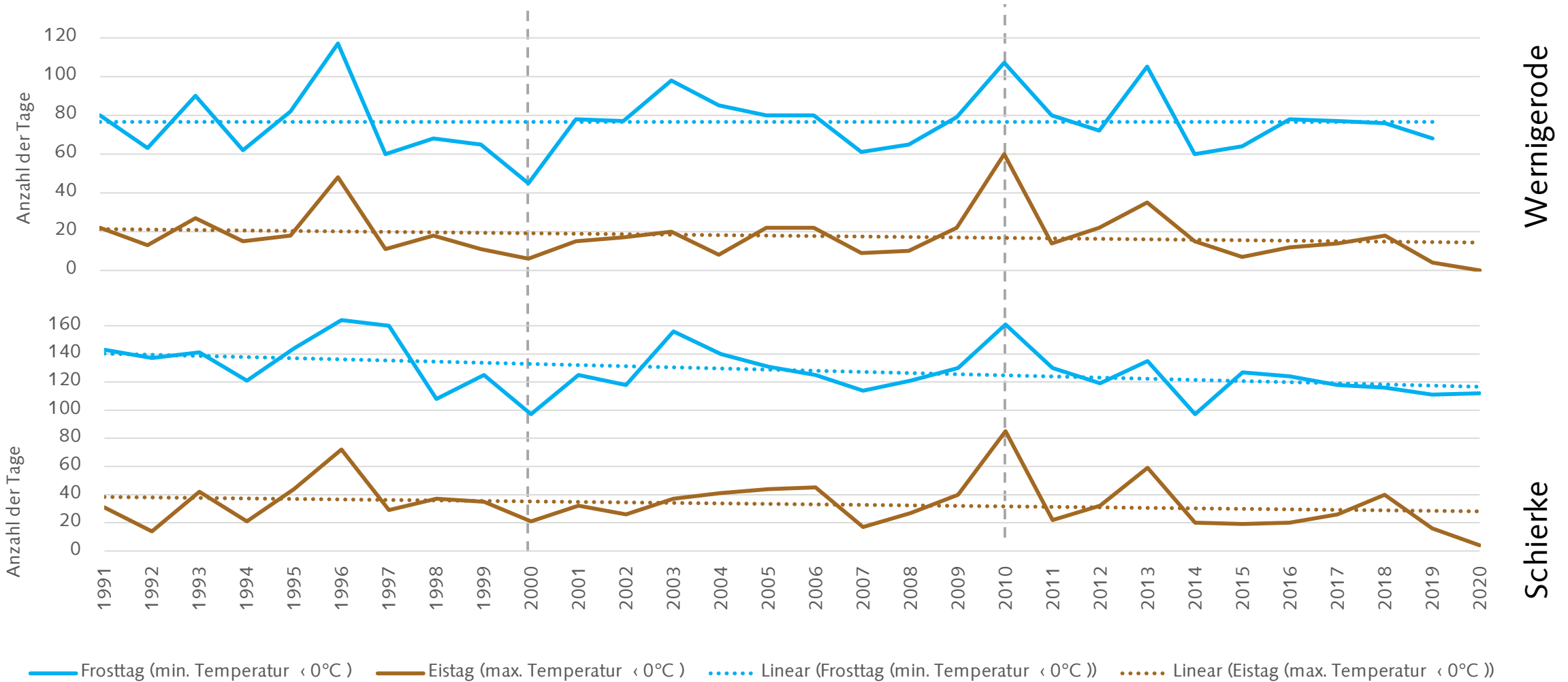
Frosttage (Tagesminimum < 0 °C) und Eistage (Tagesmaximum < 0°C)
