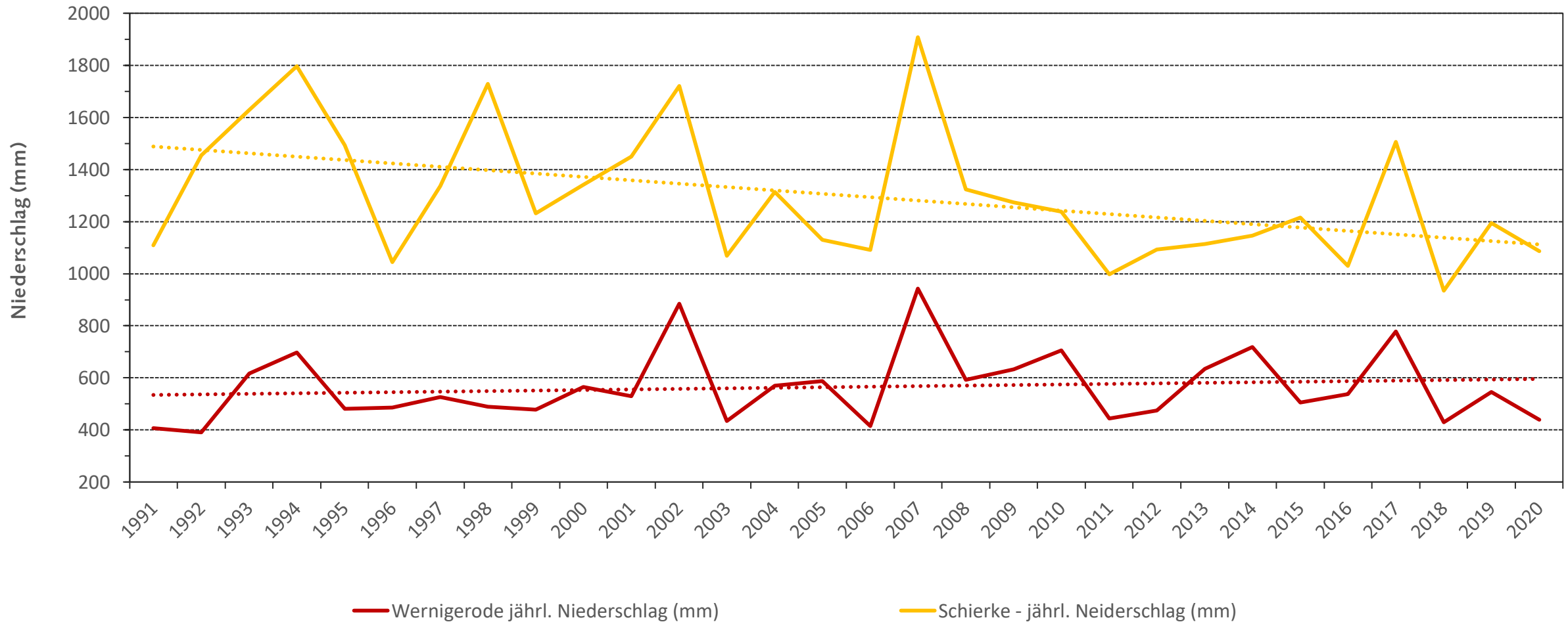
Entwicklung des jährlichen Niederschlags (mm) in Wernigerode und Schierke von 1991 bis 2020
