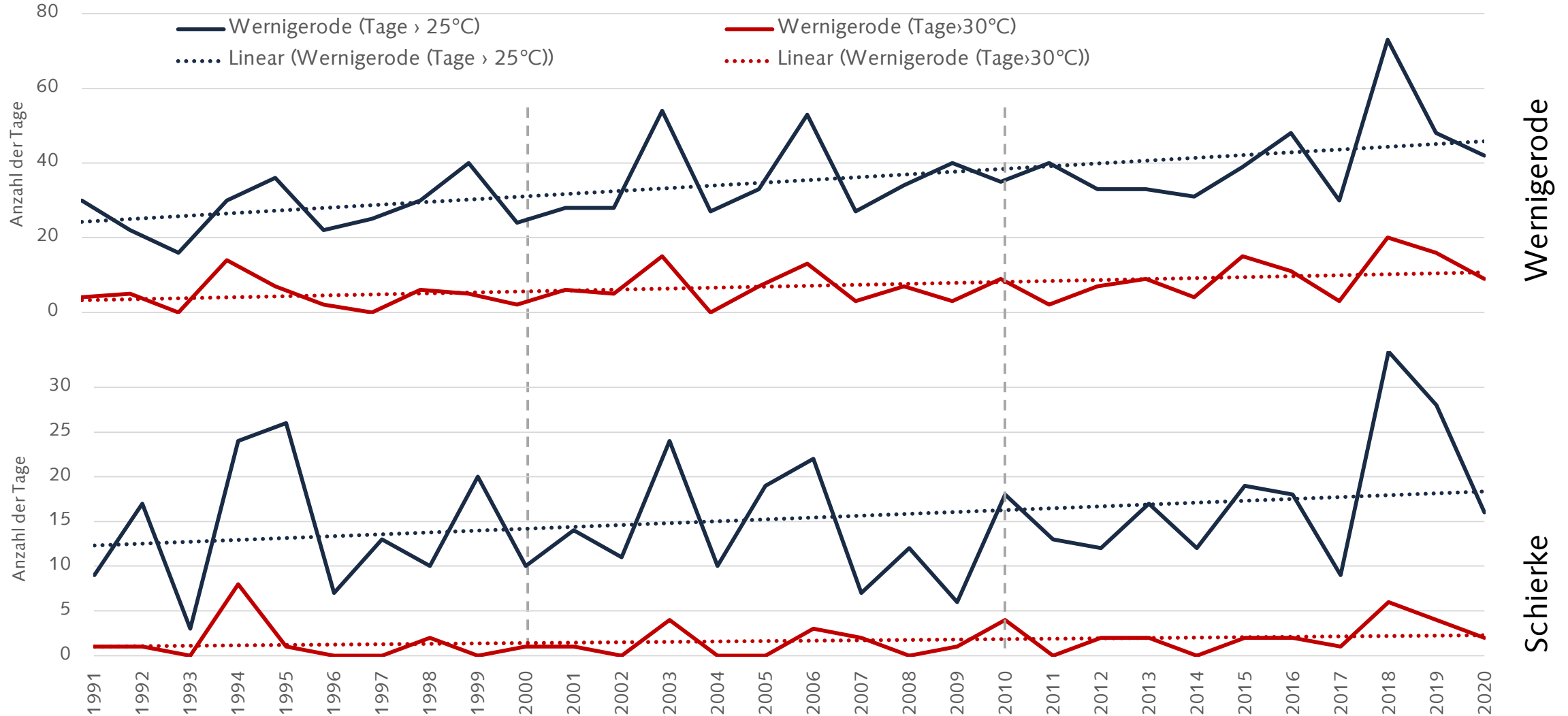
Anzahl Sommertage (> 25°C) und heiße Tage (30°C)
